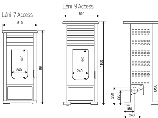
Léni 7 Access Dimensions L x H x P (cm) : 51 x 99 x 59
