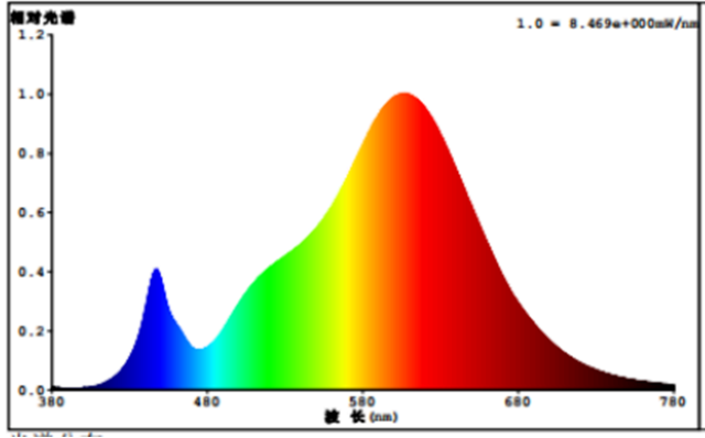
光谱参数
