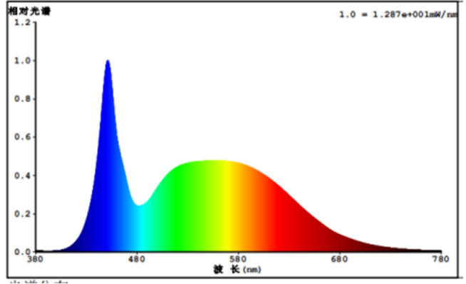
光谱参数
