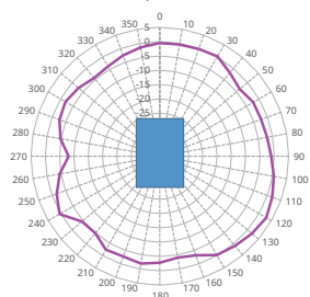
2.45G WiFi_XZ plane(antenna2,3)
