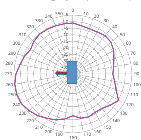
2.45G WiFi_XY plane(antenna2,3)
