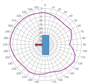
2.45G WiFi_YZ plane(antenna2,3)
