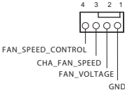
CHA_FAN1/WP
