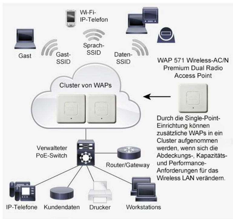
Abbildung 1. Typische Konfiguration
