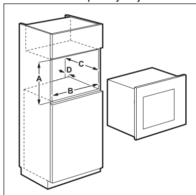
Монтажни растојанија
