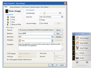
Pantalla principal de Button Manager V2
